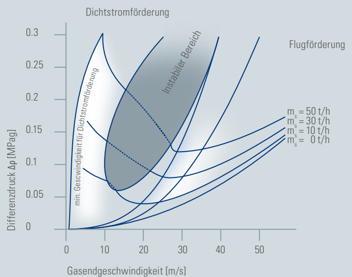
Die individuellen Zustandsdiagramme dienen der Auslegung der jeweiligen pneumatischen Fördersysteme.
